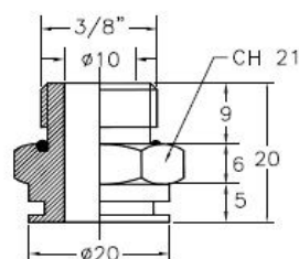
ANELLO DI RINFORZO
