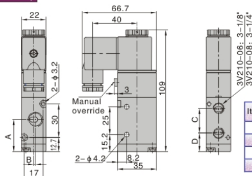
3V210(Grommet)
