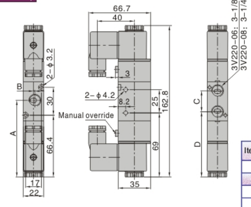
3V220(Grommet)
