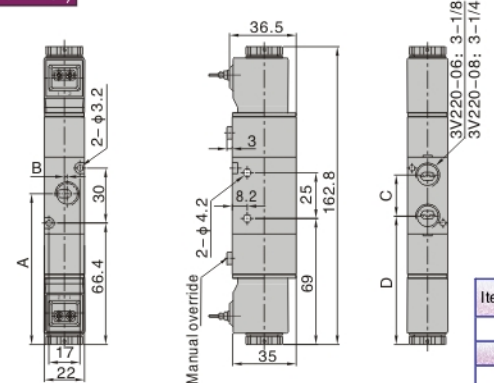
3V220(Grommet)
