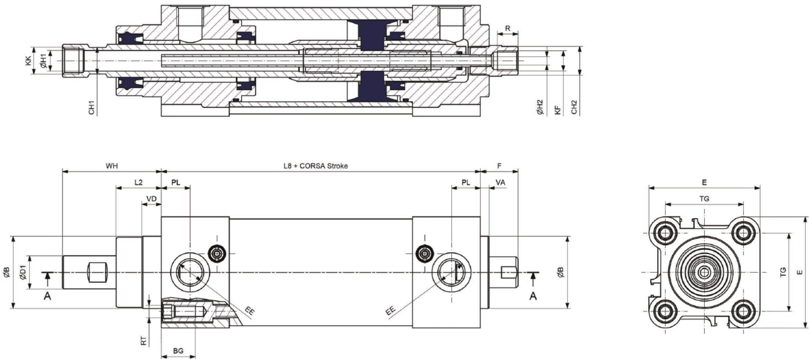
A-A (1:1)
