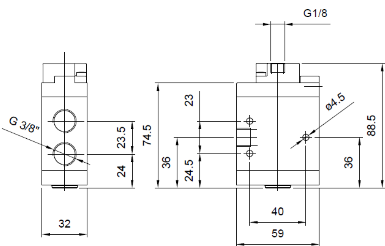
Singolo impulso pneumatico 3/8" Single pneumatic impulse 3/8"
