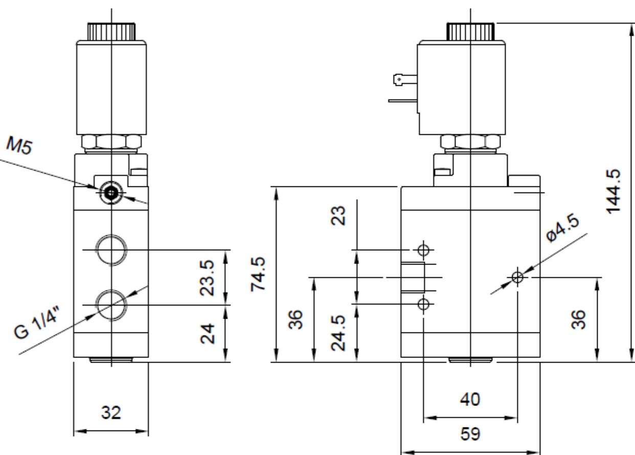
Singolo impulso elettrico 1/4" Single electric impulse 1/4"
