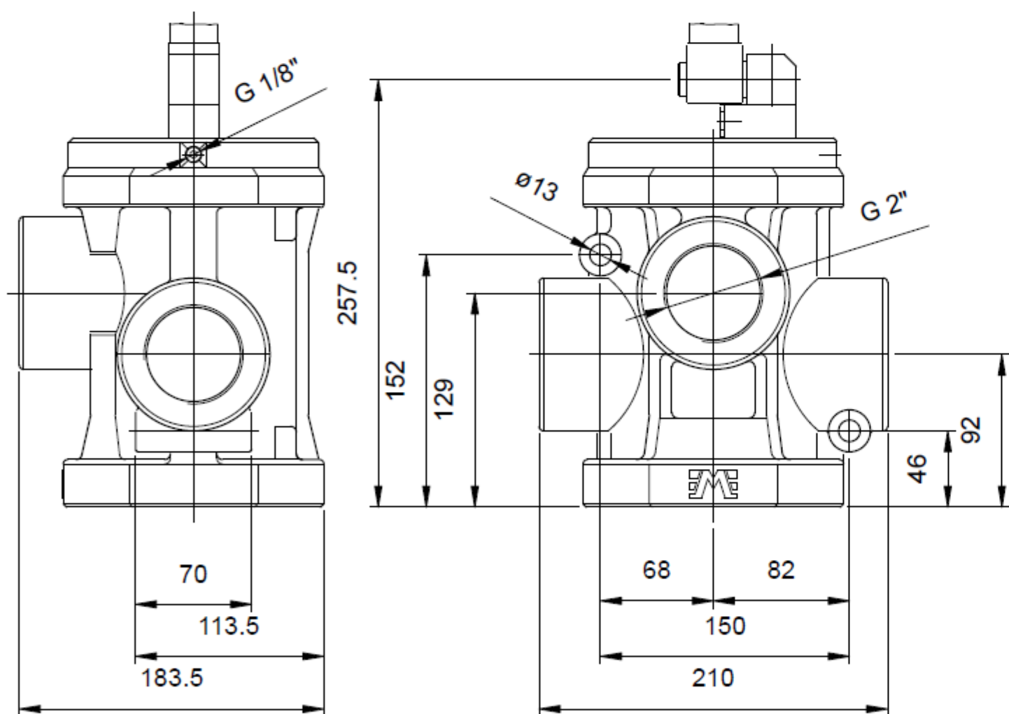
Singolo impulso elettrico 2" Single electric impulse 2"
