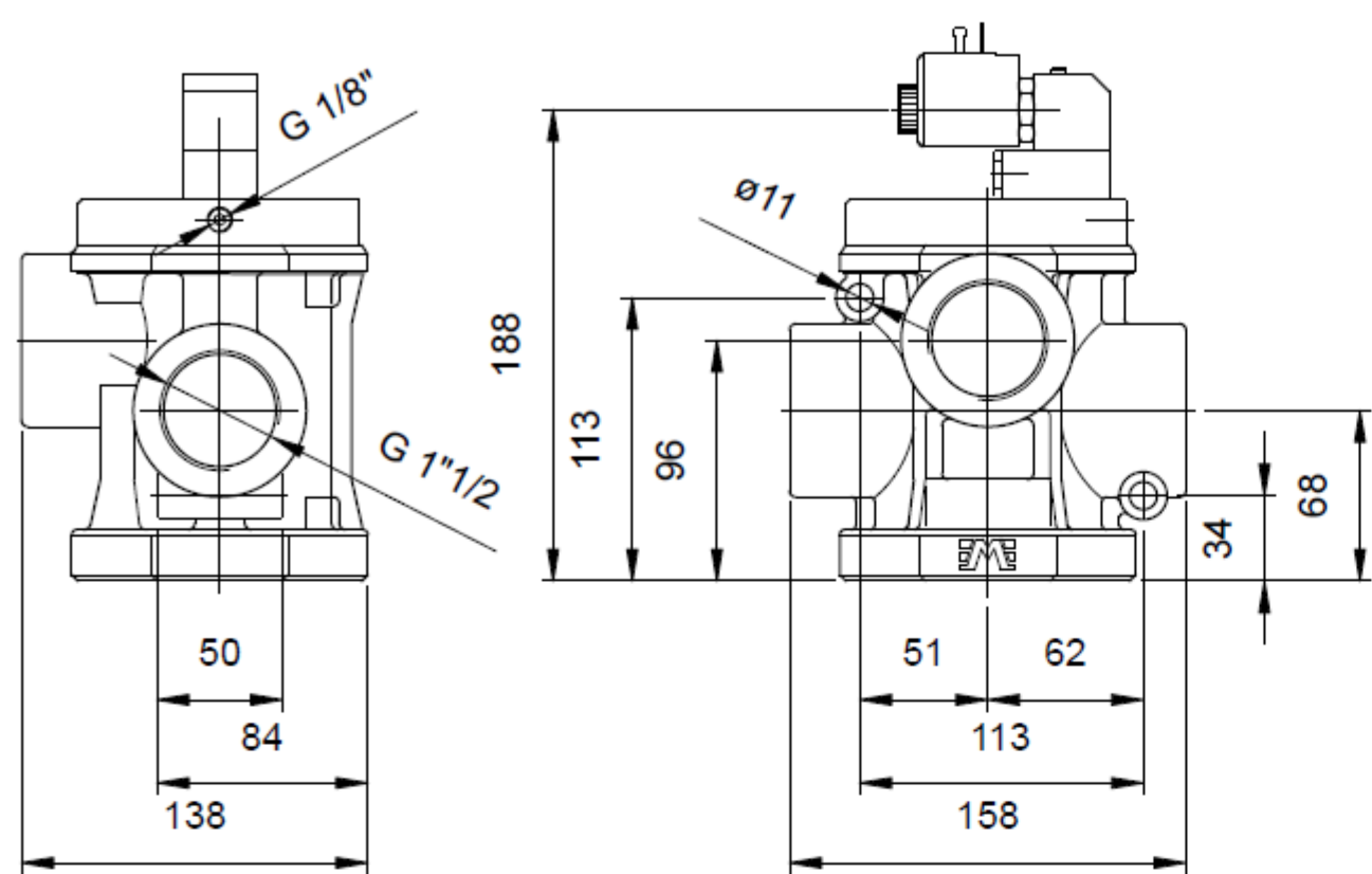
Singolo impulso elettrico 1-1/2" Single electric impulse 1-1/2"
