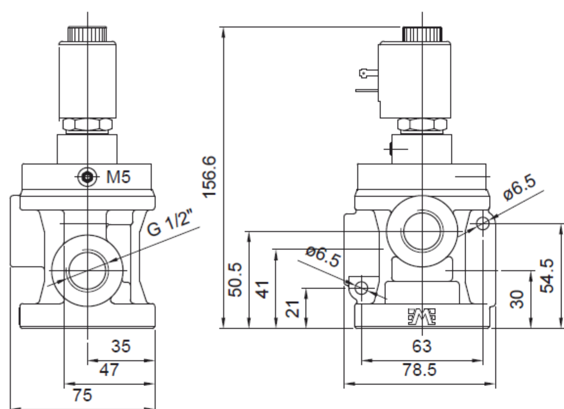
Singolo impulso elettrico 1/2" Single electric impulse 1/2"
