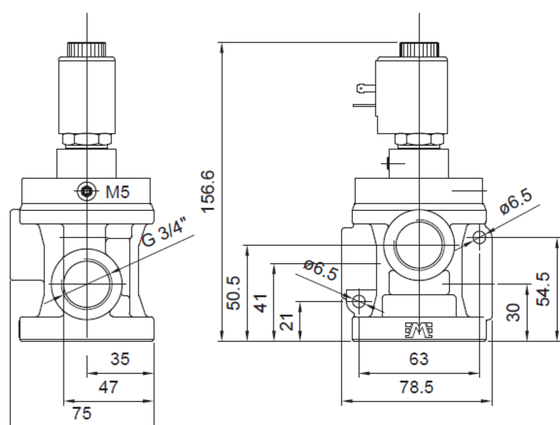
Singolo impulso elettrico 3/4" Single electric impulse 3/4"
