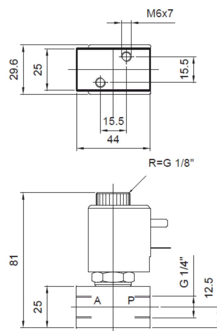
Elettropilota M2 N.C. 1/4" N.C. Electropilot M2 1/4"
