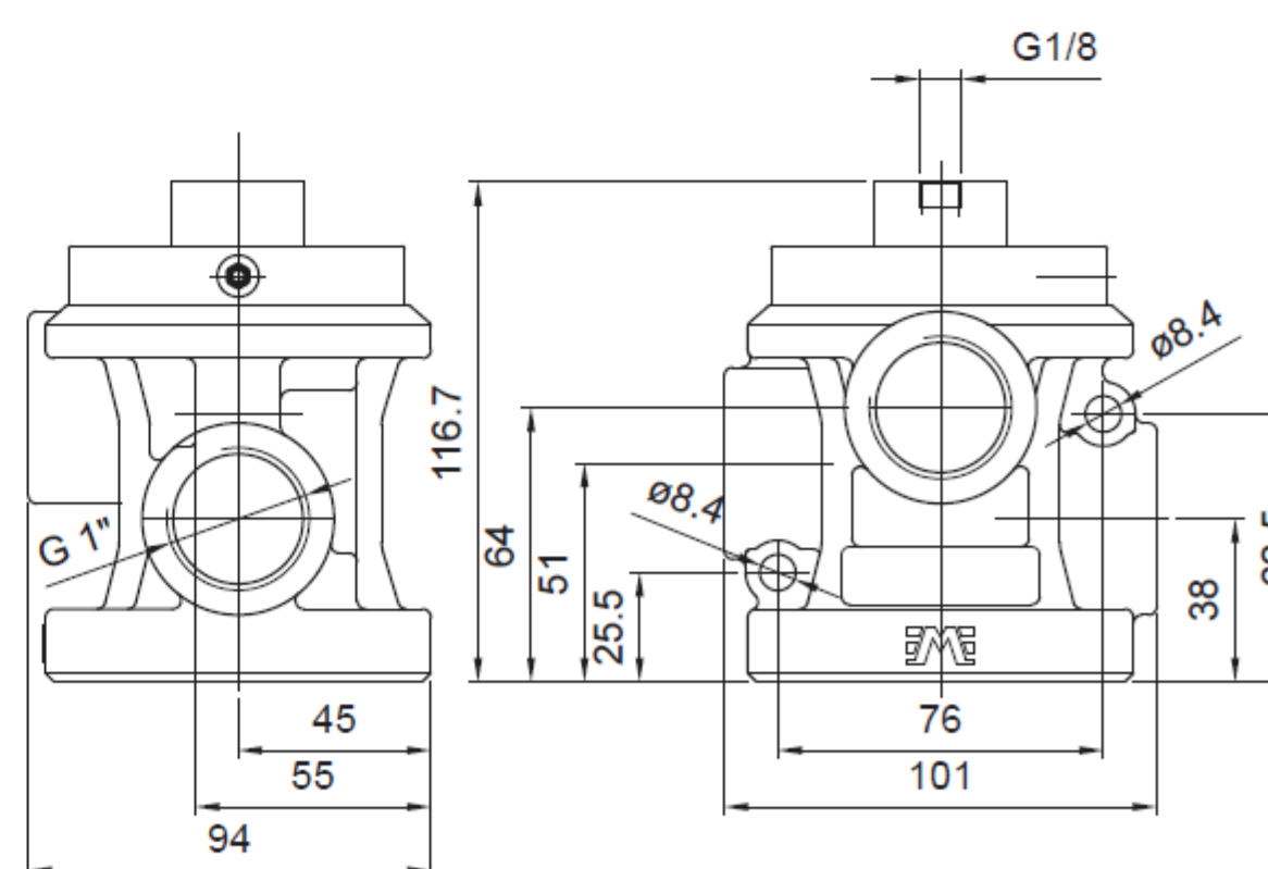
Singolo impulso pneumatico 1" Single pneumatic impulse 1"
