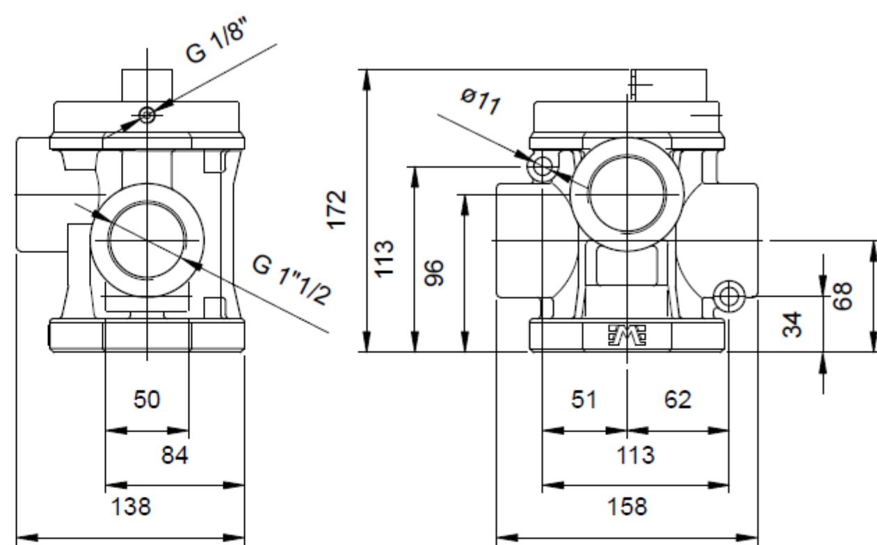
Singolo impulso pneumatico 1-1/2" Single pneumatic impulse 1-1/2"
