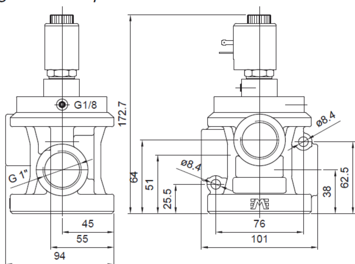
Singolo impulso elettrico 1'' Single electric impulse 1''
