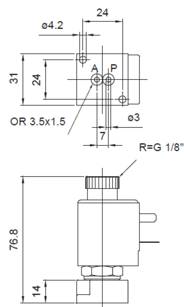
Elettropilota M2 N.A. per sottobase N.O. electropilot M2 for subbase
