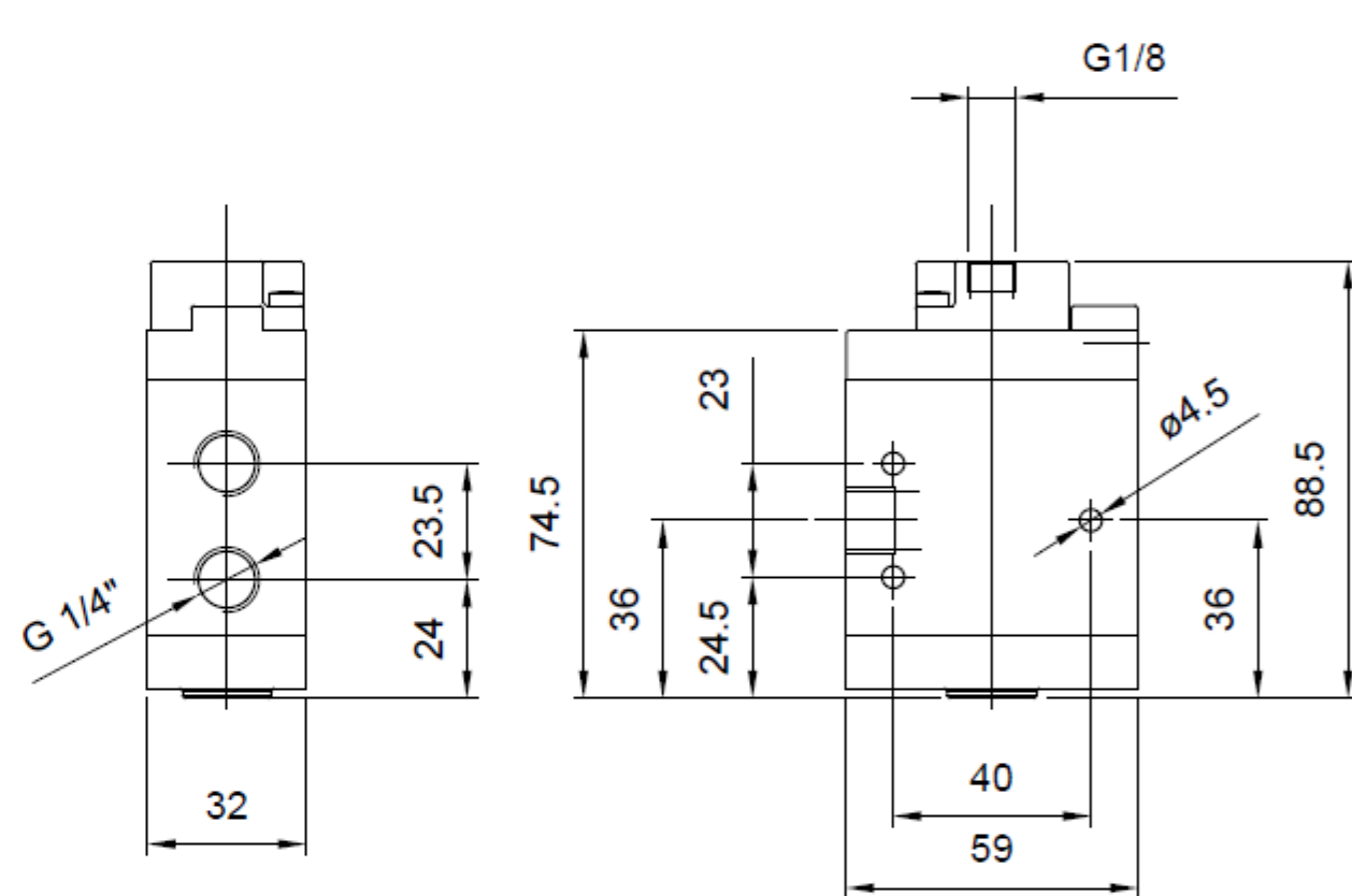
Singolo impulso pneumatico 1/4" Single pneumatic impulse 1/4"
