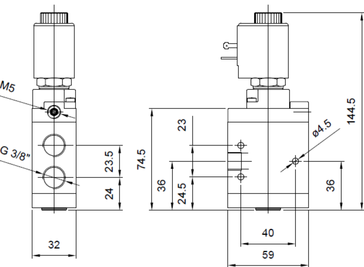
Singolo impulso elettrico 3/8" Single electric impulse 3/8"
