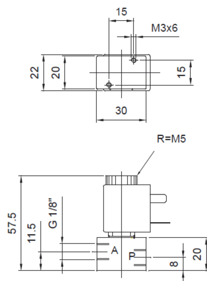
Elettropilota M1 N.C. 1/8" N.C. electropilot M1 1/8"
