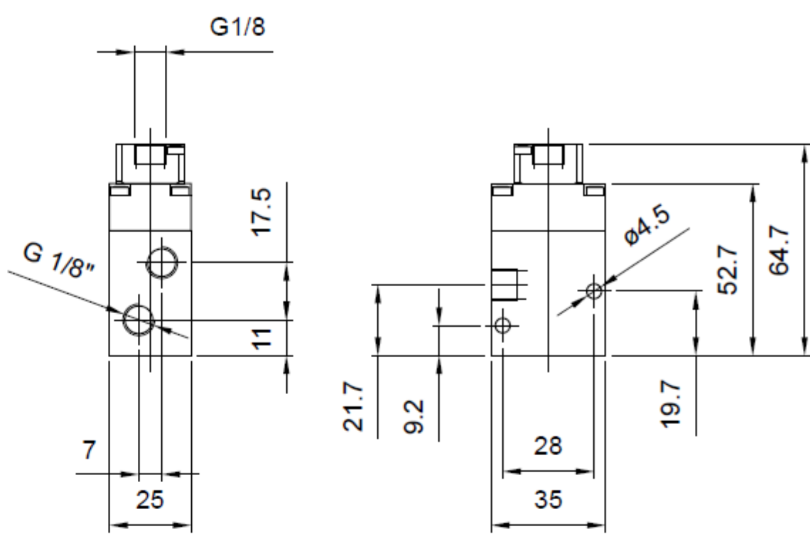
Singolo impulso pneumatico 1/8" Single pneumatic impulse 1/8"
