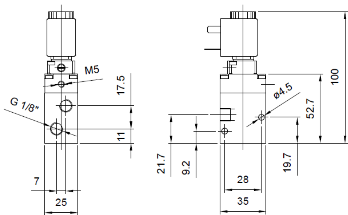
Singolo impulso elettrico 1/8" Single electric impulse 1/8"
